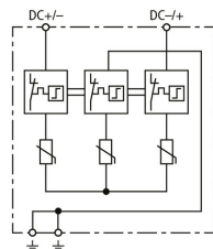
Kapcsolási rajz DCB YPV 1500
